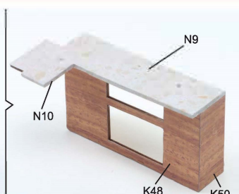
19 Sklej drewniane elementy jak na zdjęciu. Przyklej papier.
