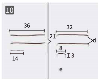
10 Potnij i zagnij drut jak na zdjęciu.
