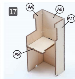
17 Sklej drewniane elementy jak na zdjęciu.
