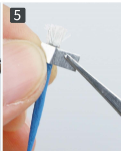
5 Zawiń folię alu. jak na zdjęciu.
