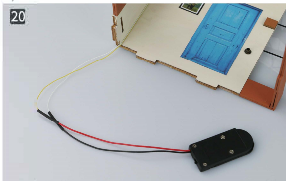
20 Połącz przewody lampy z przewodami obudowy. (żółty z czerwonym, biały z czarnym) Zgrzej rurki zapalniczką.
