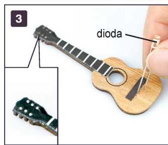
Zrób otwory zgodnie z M11 i M6. (użyj nóżek diody)
