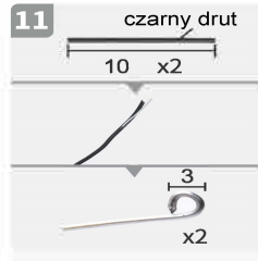
Potnij drut. Usuń izolację i zagnij jak na zdjęciu.
