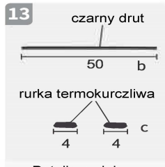
Potnij zgodnie ze zdjęciem.
