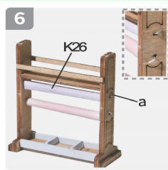
Wykonaj w ten sam sposób, zagnij końce.
