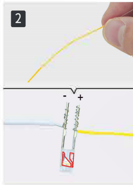
2 Usuń izolację z przewodów(12mm).Połącz żółty z anodą(+),biały z katodą(-).
