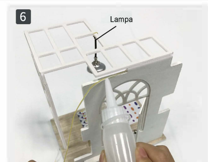
Przyklej lampę oraz przewód jak na zdjęciu.
