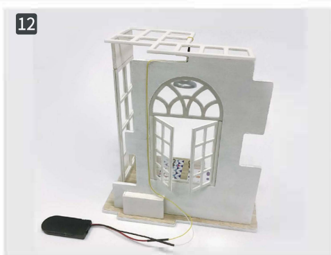
Połącz przewody lampy z przewodami obudowy baterii (żółty-czerwony, biały-czarny). Wykonaj test po połączeniu. Zgrzej rurki termokurczliwe zapalniczką.
