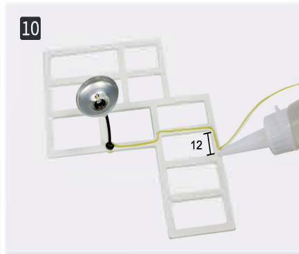
10 Przyklej przewód jak na zdjęciu,zachowaj odstęp od krawędzi.
