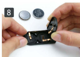
Umieść baterie w obudowie (zwróć uwagę na + i -).
