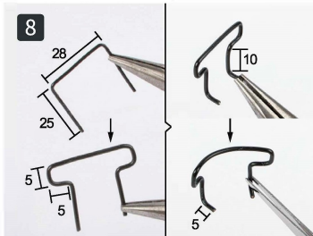
Zagnij drut jak na zdjęciu.
