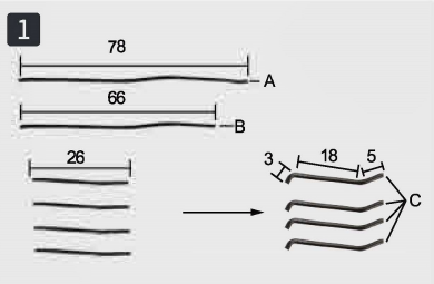
Potnij i zagnij drut jak na zdjęciu.
