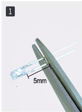
1 Ostrożnie utnij diodę jak na zdjęciu.
