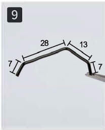
Zagnij odcinek D jak na zdjęciu.
