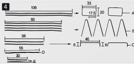
Potnij i zagnij drut jak na zdjęciu.
