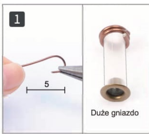
Zgnij drut i owiń rurkę jak na zdjęciu.
