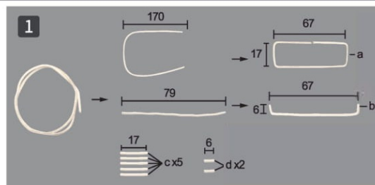
Potnij i zgnij drut pęsetą jak na zdjęciu.
