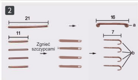
Potnij i zgnij drut jak na zdjęciu.
