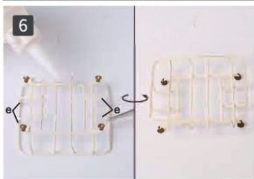
Przyklej drut e na spodzie bagażnika.
