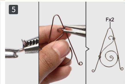
5 Zagnij E jak na zdjęciu, następnie połącz z A,B jak na zdjęciu. Wykonaj 2 szt. F.
