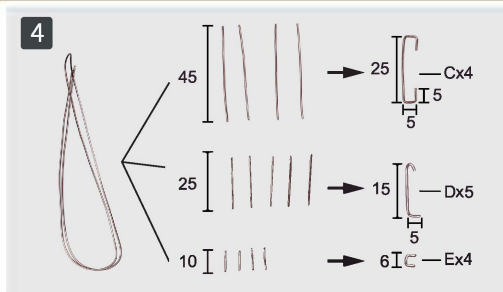
4 Potnij i zagnij cały drut jak na zdjęciu.
