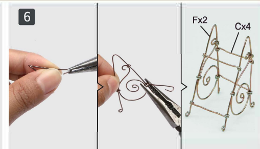
6 Zagnij C jak na zdjęciu, następnie połącz z F(2szt.) jak na zdjęciu.
